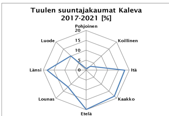
Kuva 5. Tuulen suuntien tuntikeskiarvojen prosenttijakaumat Kalevan mittausasemalla vuosina 2017–2021 tuuliruusuna.
